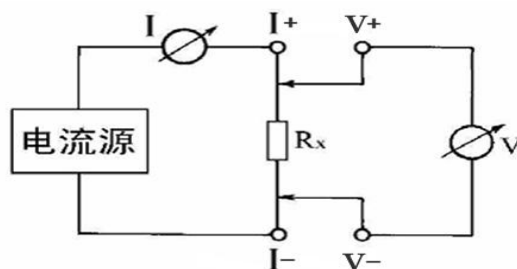
图二 测试原理图
