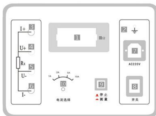
图一 面板布局图
