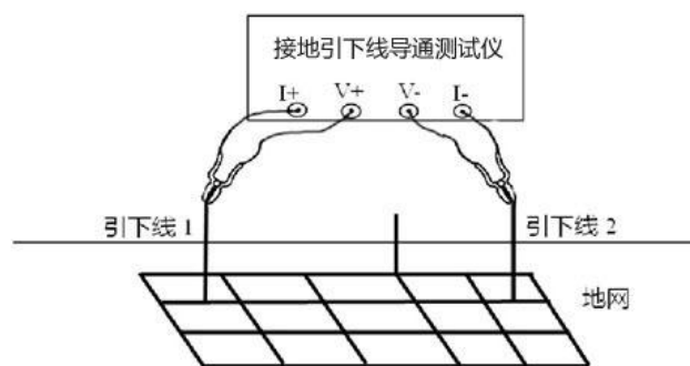
图三 四端子接线图
